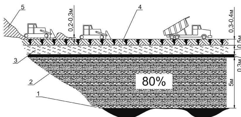
Rys. 4. Schemat technologiczny górnictwa-technicznej rekultywacji wyrobiska (opracowanie własne)
